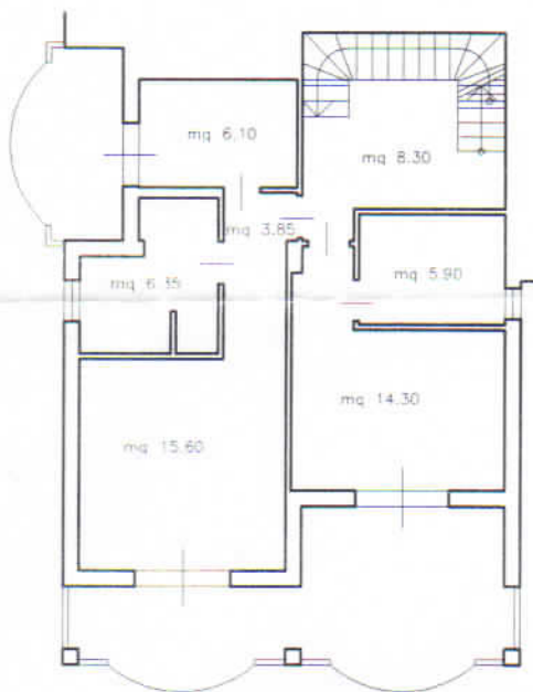
PIANO PRIMO
